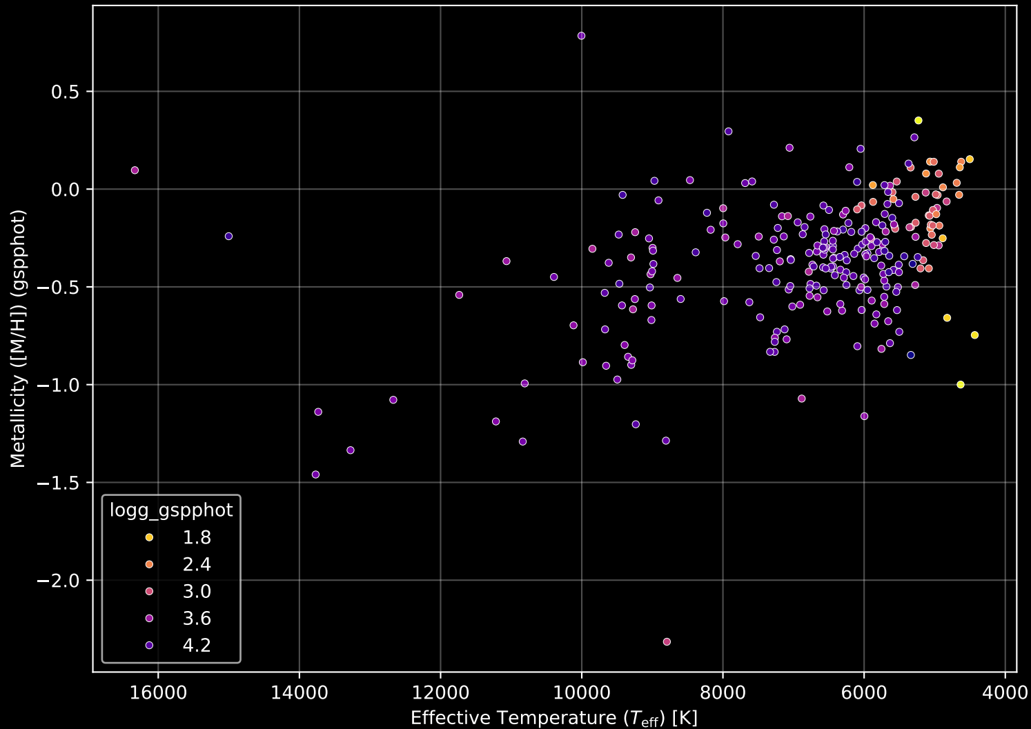
GALAH DR4 Field: [9276] Stellar Population Parameters (n= 267)
