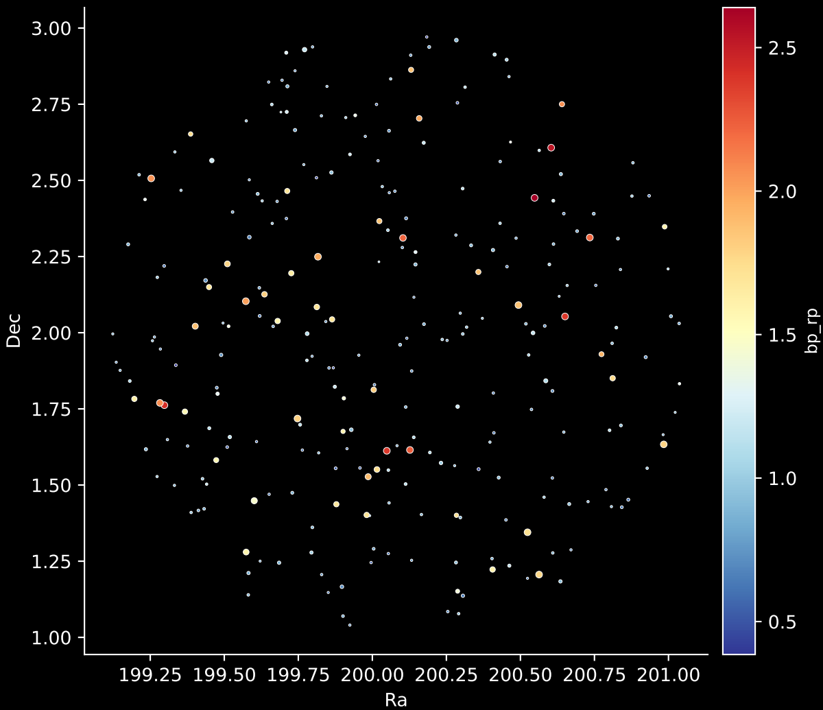
GALAH DR4 Field: [9276] Stars: 267
