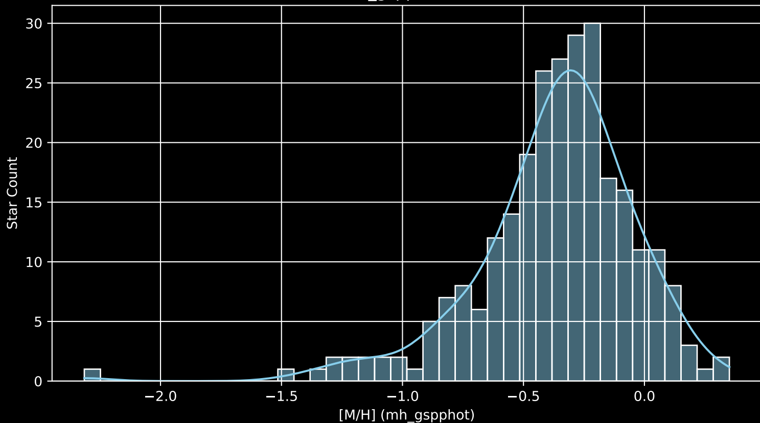
GALAH DR4 Field: [9276] [M/H] (mh_gspphot) (n= 266)
