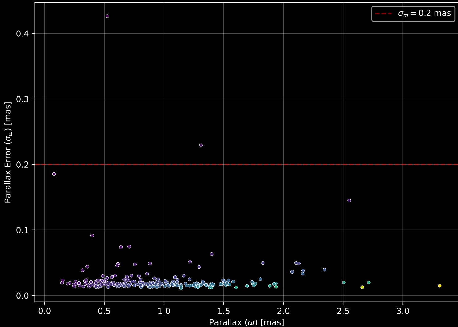
GALAH DR4 Field: [9276] Parallax Quality (n= 267)
